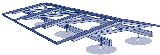
Ost-West-Anlage (10° Neigung)
