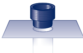
EPDM-Anstauring EPDM, höhenvariabler Anstauring Innen-Ø 75/110/125/160 mm
