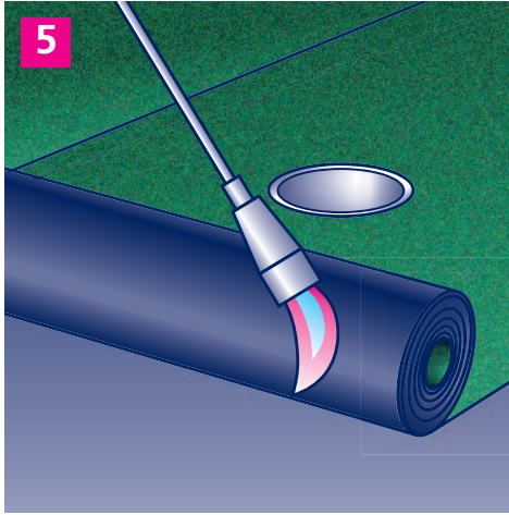
5. Oberlage im Bereich des Grundelements ausschneiden, danach aufschweißen bzw. aufkleben.
