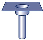
Topf-Gully senkrecht Edelstahl, ohne Wärmedämmung Ø 75/110 mm
