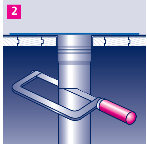
2. Bei Bedarf kann der Stutzen des Grundlements mit langem Stutzen gekürzt werden. Dabei ist die Mindesteinstecktiefe der Muffe des Anschlussrohrs zu beachten!
