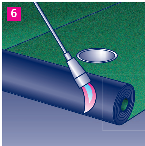
6. Oberlage im Bereich des Grundelements ausschneiden, danach aufschweißen bzw. aufkleben.
