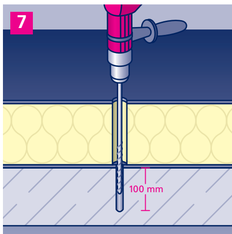
7. Konzentrisch zum Ausschnitt in der Dämmung ein Loch ( \varnothing 10 mm, mind. 100 mm tief) für das Einsetzen des Betonankers bohren. Als Zentrierhilfe nutzen Sie ggf. den umgedrehten Lochschneider.
