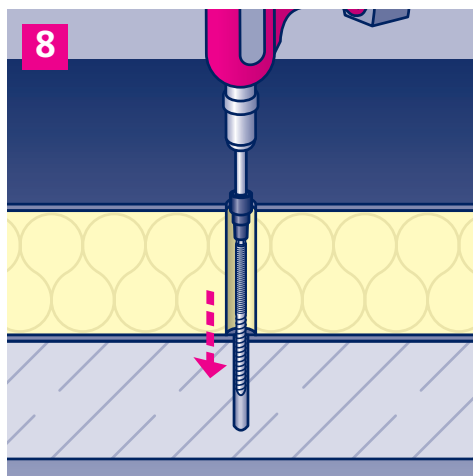
8. Bohrloch durch Aussaugen oder -bürsten säubern. Dann den Betonanker mit Hilfe des Konsolenankers SMART ( \varnothing 8 mm, 1/2") 80 mm tief in den Beton drehen.
